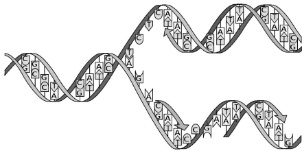
Bij de replicatie bewegen de twee strengen van het DNA uit elkaar om te worden gekopieerd. Bron: Wikipedia
