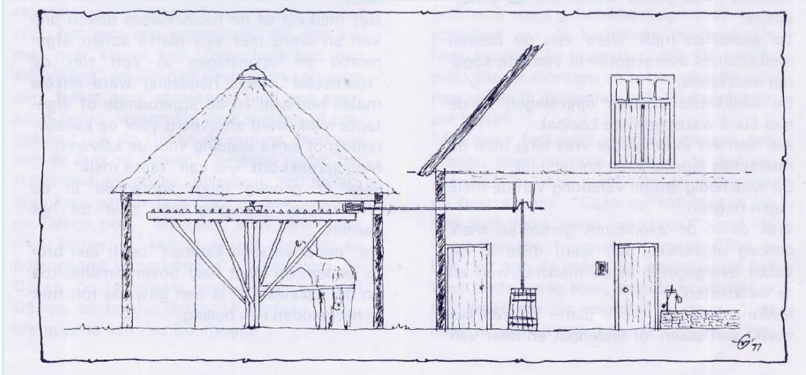
Een doorsnede van een karnmolen en het achterhuis met de karnton en de koelbak
