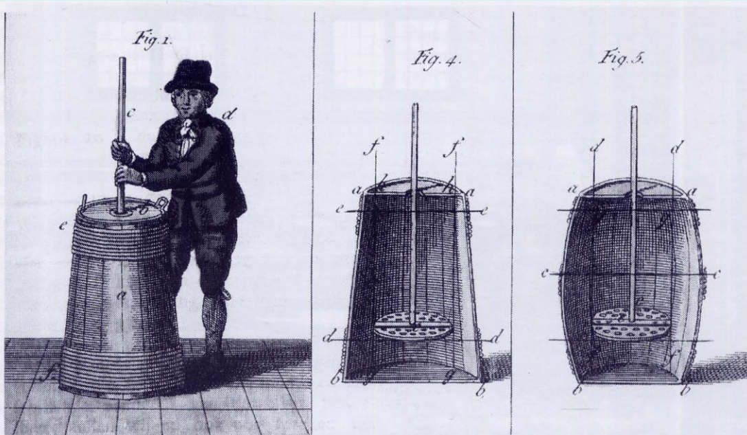
Het karnen met de hand bij een ouderwetse karnton. De doorsnede laat de karnstok zien met de ronde plank met gaten, "de druif".
