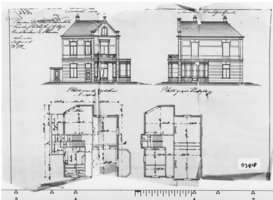
Figuur 7 Tekening van Villa Arti met de namen van de opdrachtgever en de architect. Coll. AGV
